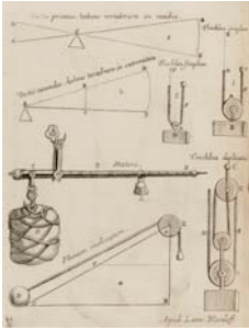
Blendeff 19 Vectis, statera, trochlea, planum inclinatum (ms. 211, fol. 259v)
