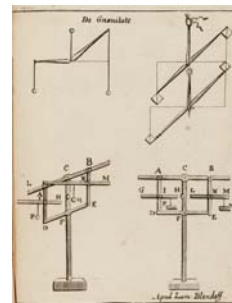
Blendeff 18 De gravitate (4 voorbeelden van evenwicht) (ms. 211, fol. 258)
