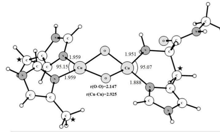
3(d) – Bis-oxo -3A
