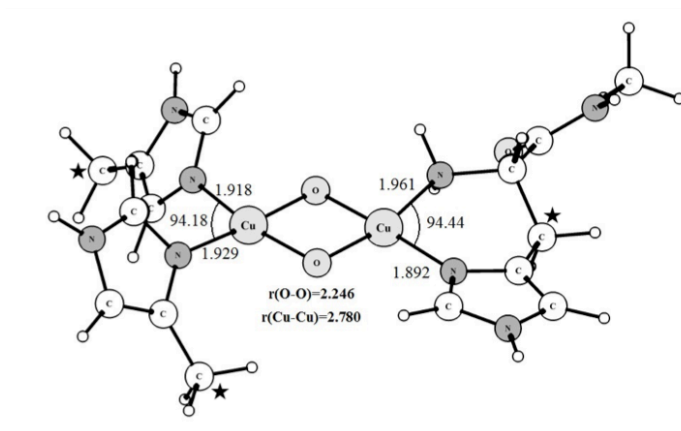
3(c) – Bis-oxo -1A
