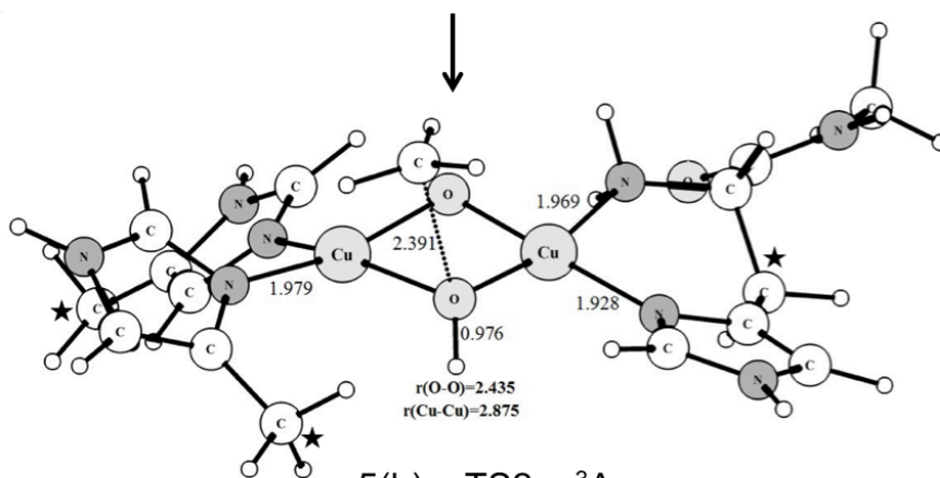
5(b) – TS2 – 3 A
